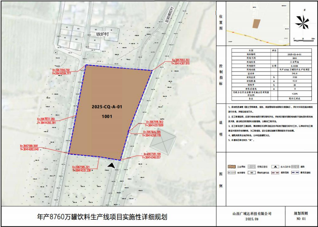
附件：用地规划图
